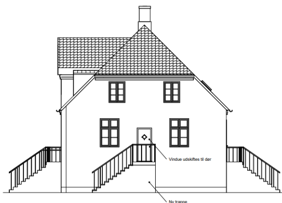
Nordfacade
