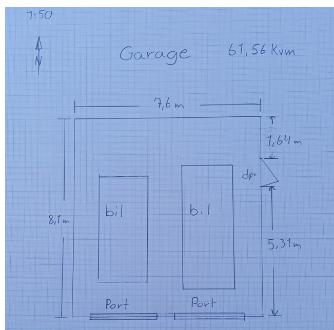
Figur 3 Tegning af den ønskede garage hentet fra ansøgningen.
