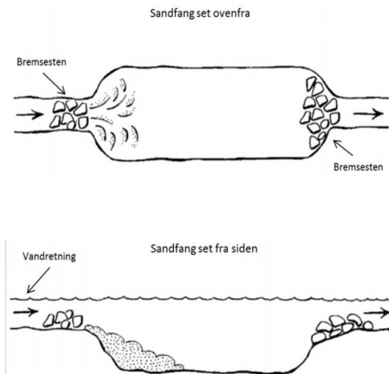
Fig 2.: Her vises et generisk sandfang. Hvor Ind- og udløb sikres med sten og på udløbssiden lægges der desuden en strækning med grus, til at sikre sandfanget ikke afgiver uønsket materiale til nedstrømsliggende arealer. Desuden har gruset en beskaffenhed der gør det egnet som gydeområde for ørreder. Derved opnår man en yderligere positiv effekt af sandfangets etablering.
