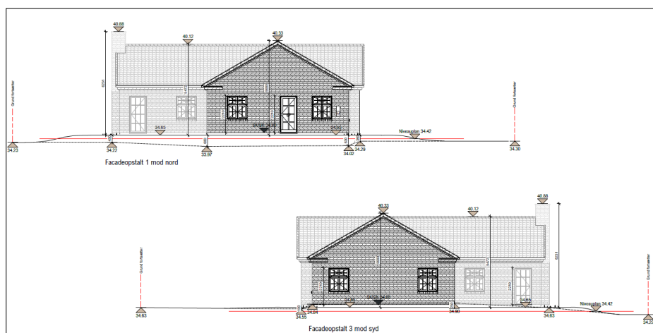
Fra ansøgningen: Tegninger af facader mod nord og syd
