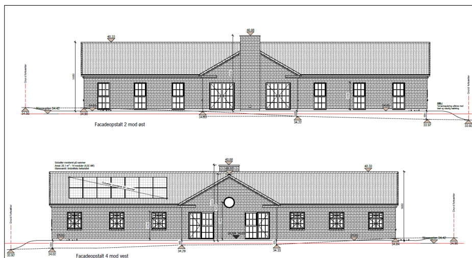
Fra ansøgningen: Tegninger af facader mod øst og vest
