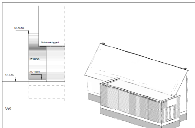
Fra ansøgningen: Facade mod syd og et 3D-model af den ansøgte bygning
