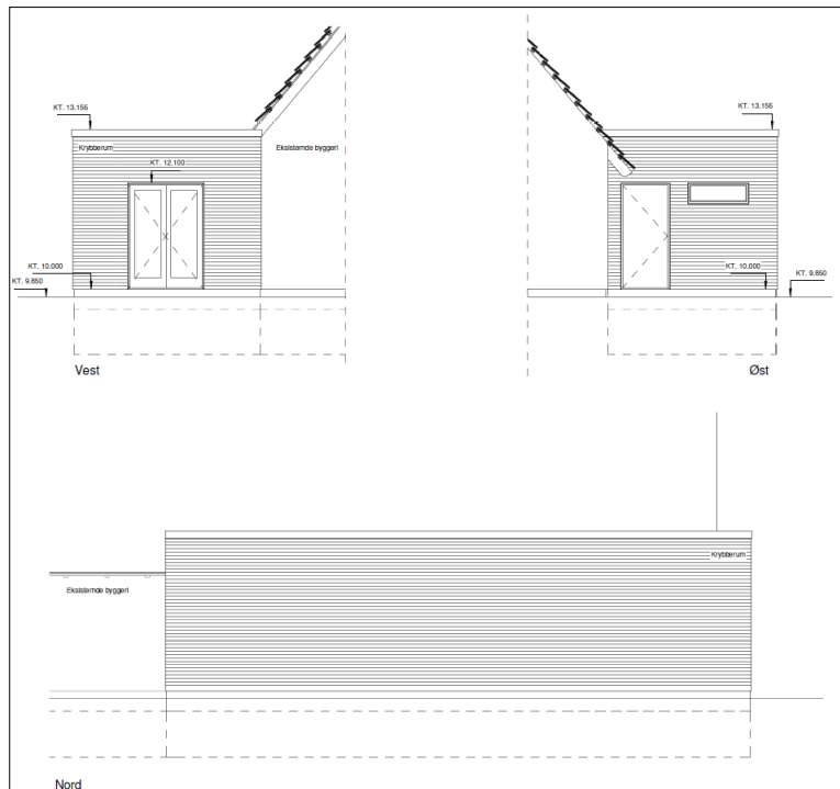
Fra ansøgningen: Facaderne mod vest, øst og nord
