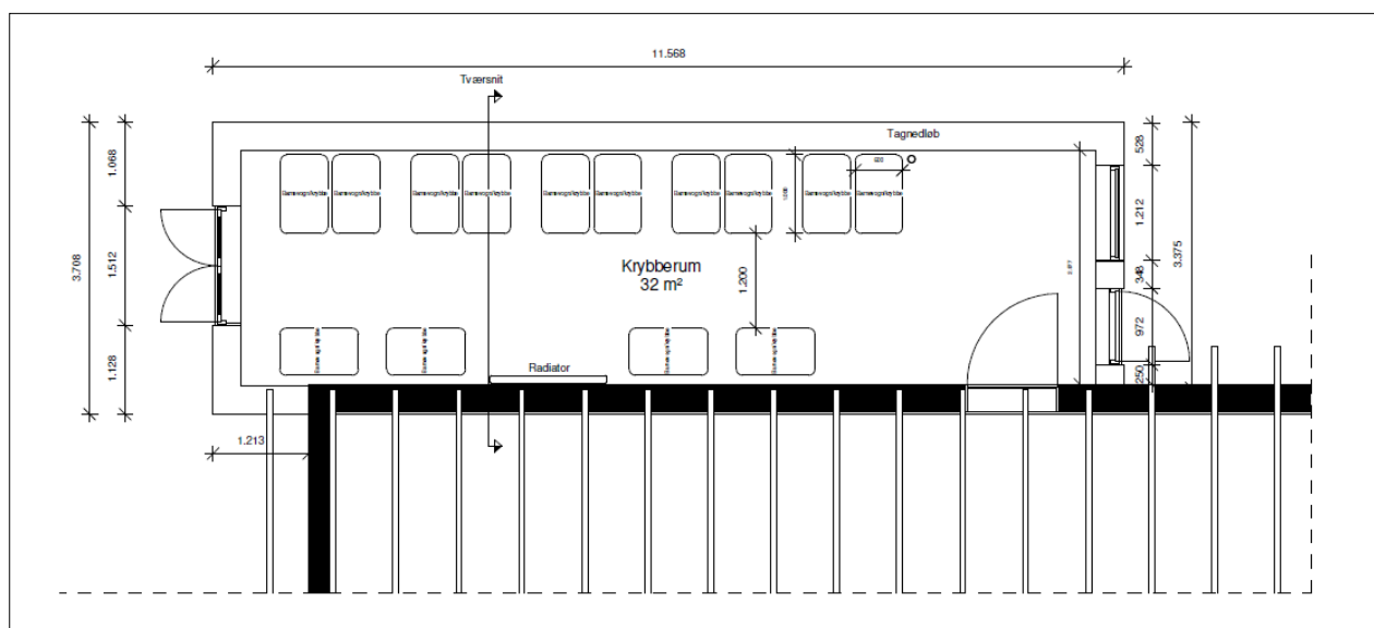
Fra ansøgningen: Plantegning
