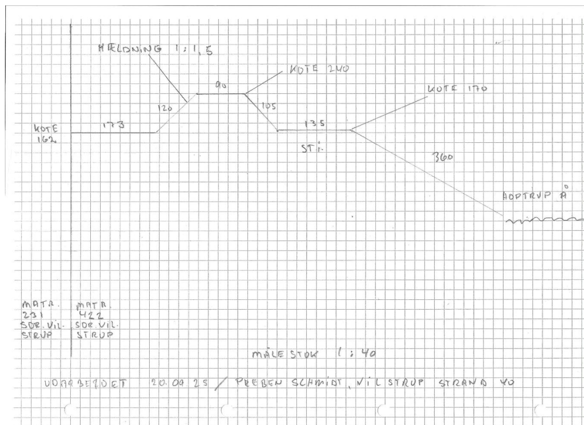
Figur 3: Illustration af det endelige tværsnit, hvor der er angivet en hældning på ådigets bagside. Ådiget bagside går fra kote 240 til 162 meter over daglig vande og har dermed en hældning på 1:1,5.
