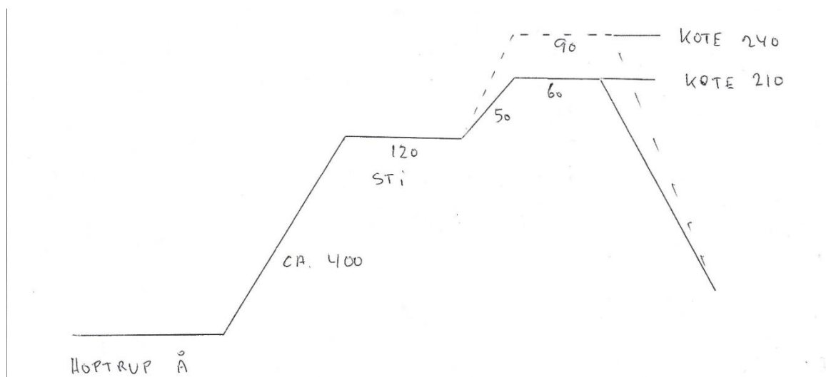
Figur 1: Første tværsnittet fremsendt i ansøgningen.
