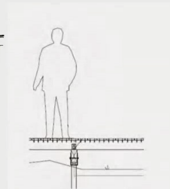
Principskitse af opbygningen af en boardwalk, der er hævet op over terrænet for at skåne underlag og natur mindst muligt.
