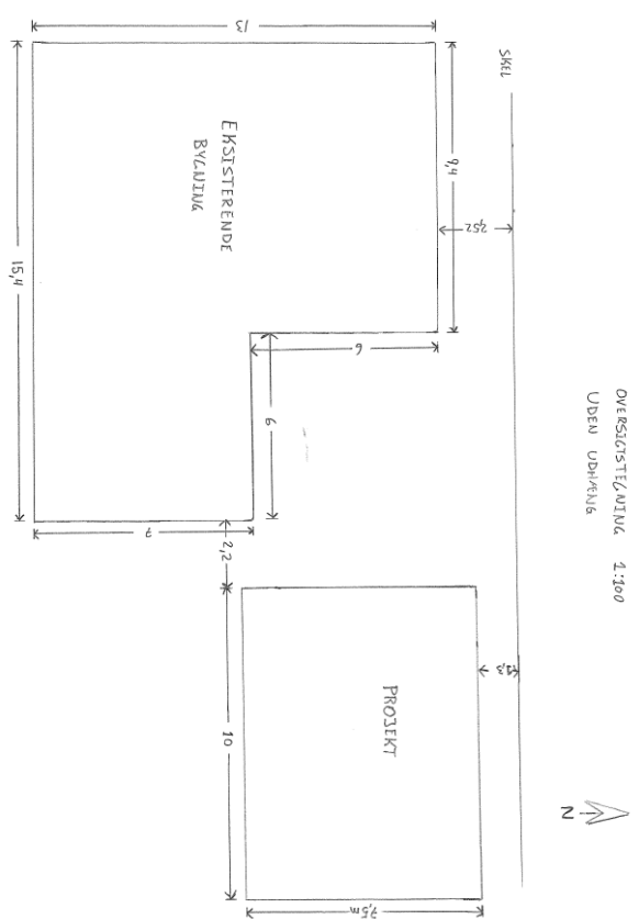
Figur 3 Oversigtstegning fra ansøgning. Bebyggelsen er vist uden udhæng
