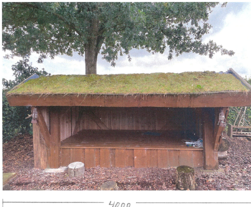
Figur 15 Foto fra ansøgning af shelter set forfra og med angivelse af mål
