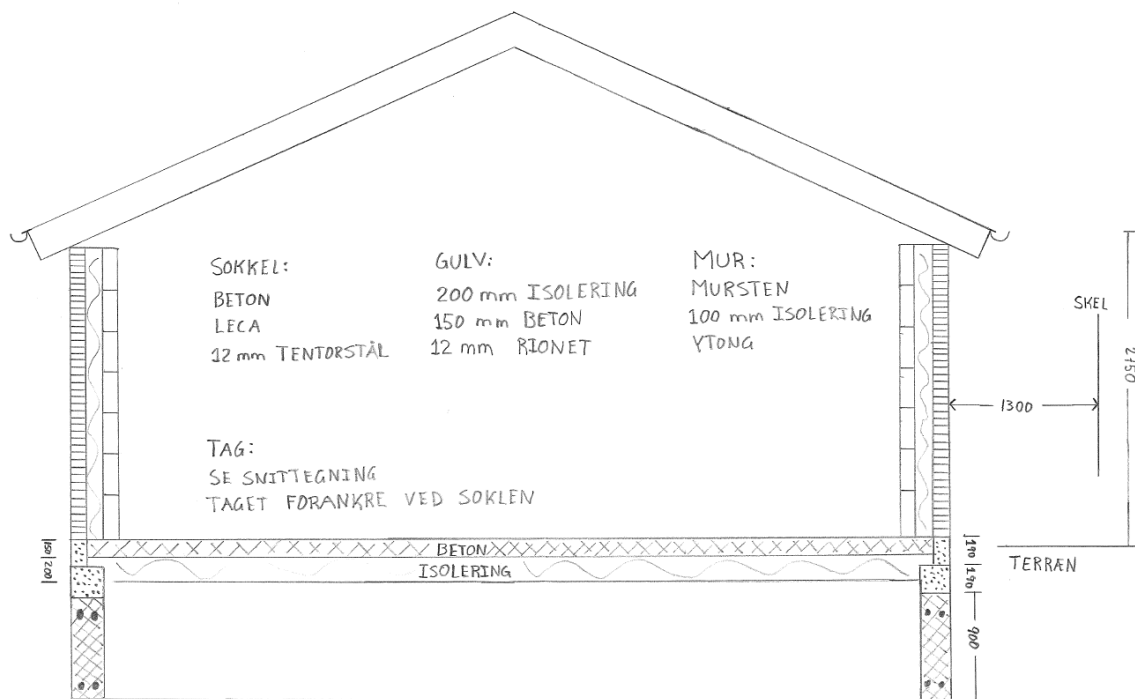
Figur 13 Snittegning fra ansøgning incl. materialer
