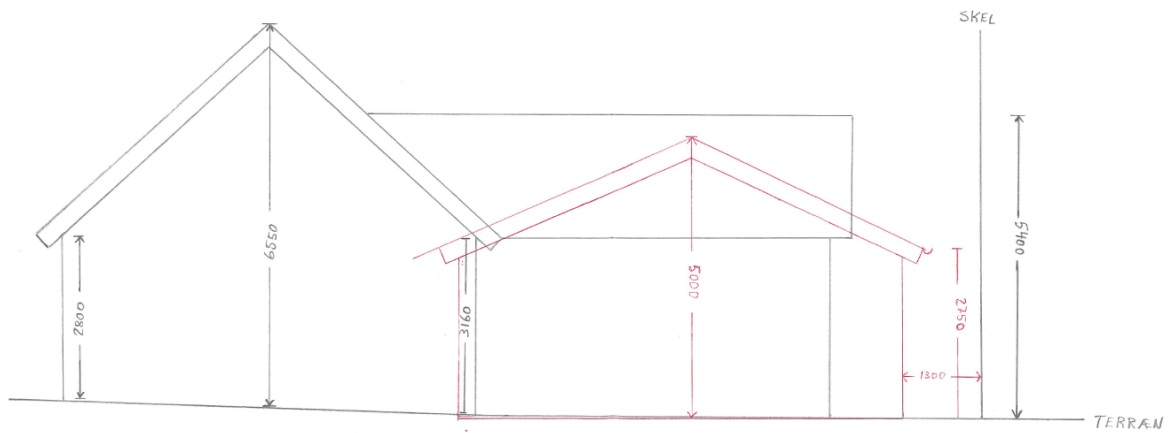
Figur 9 Snittegning fra ansøgningen. Bebyggelsen set fra øst mod vest
