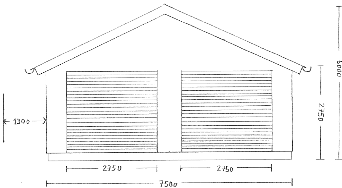
Figur 10 Snittegning set fra vest mod øst
