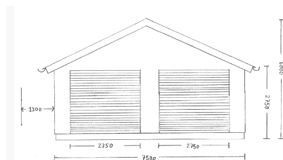
Figur 4 Snittegning fra ansøgningen der viser garagen set fra vest mod øst
