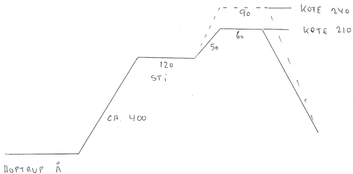
Bilag 1: Tværsnit af dige.
