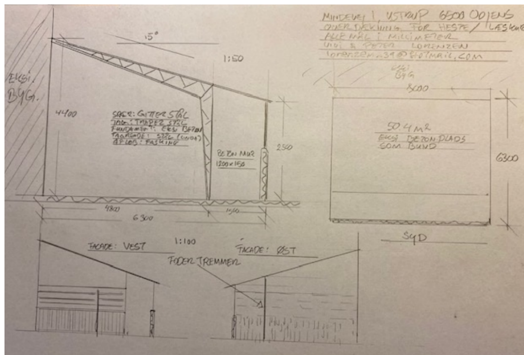
Fra ansøgningen: Plantegning, facadetegninger og snit
