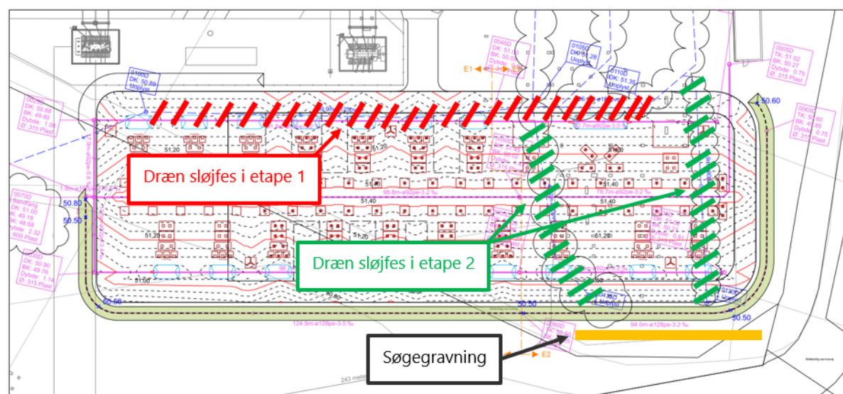
Figur4: Dræn, der sløjfes i etape 1, er vist med rød markering. Dræn, der sløjfes i etape 2, er vist med grøn markering. Den orange linje angiver søgegravning efter udefrakommende dræn.
