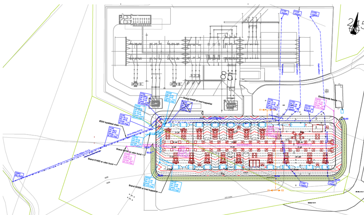
Figur 3: Eksisterende drænledning og udløb er indmålt samt indtegnet som blå stiplede linjer
