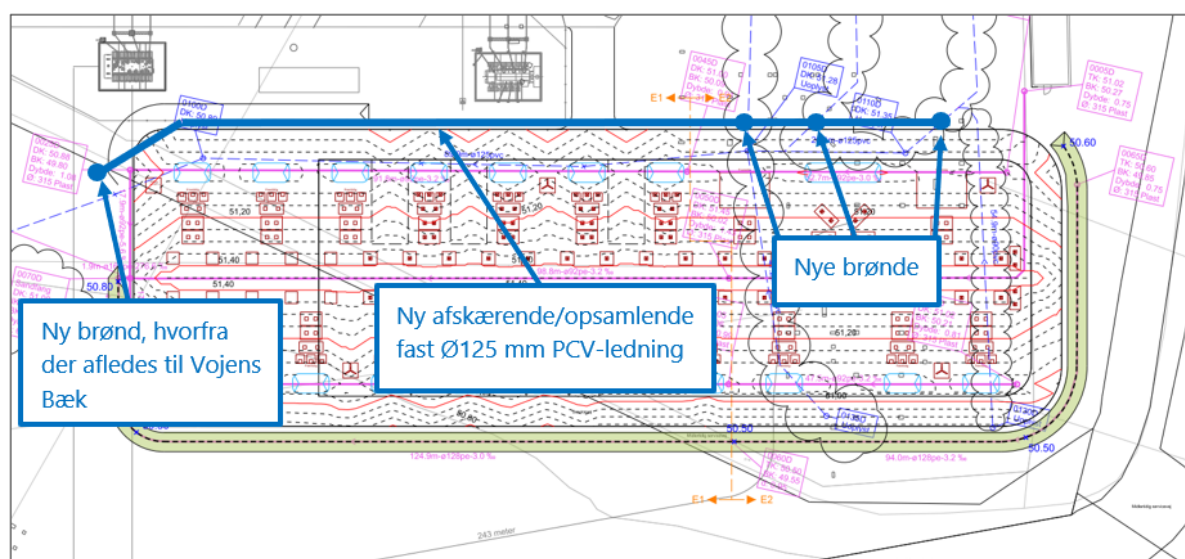
Figur 5: Ny afskærende/opsamlende fast Ø125 mm PVC-ledning samt nye brønde er angivet med blåt.
