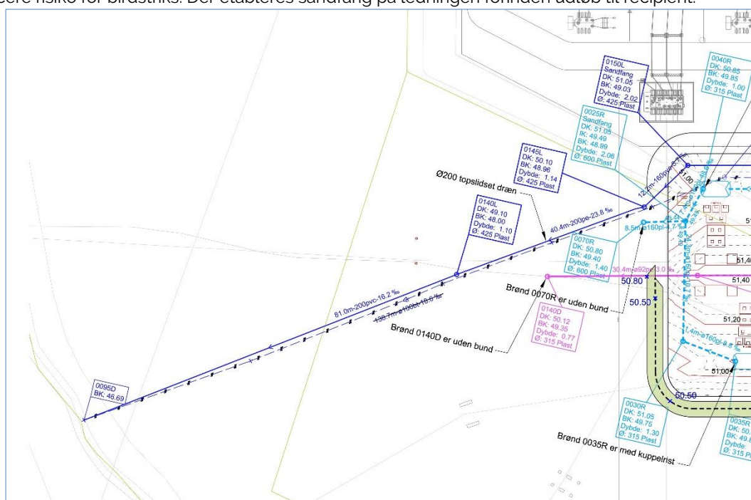
Figur 6: Omlægning af eksisterende Ø100 mm betonrørledning til fast Ø200 mm PVC-rørledning.
