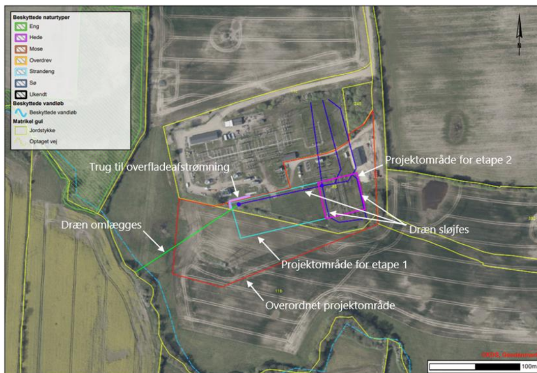
Figur 2: De blå linjer markerer eksisterende dræn i området. Det turkise rektangel markerer omrids af den nye transformatorstation i etape 1. Den lyserøde firkant markerer omrids af etape 2. Den lilla linje markerer trug til styring af overfladeafstrømning (truget bliver delvis beliggende på matrikel 11c Maugstrup Ejerlav, Maugstrup). Den grønne linje markerer rørledning til Vojens Bæk, der omlægges. Beskyttede naturtyper er vist med signaturforklaring i øverste venstre hjørne. Bemærk at signatur for § 3-beskyttet vandløb er forskubbet ift. det reelle forløb af Vojens Bæk. De gule streger angiver matrikelskel.
