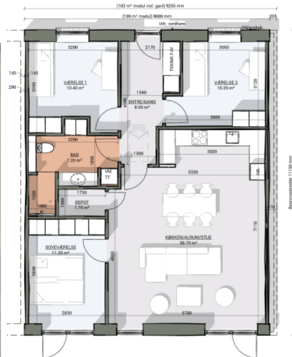
Tegning af hus fra ansøgning Hustype: Længe hus 101,0 m 2 Tagtype: Saddeltag/valmtag
