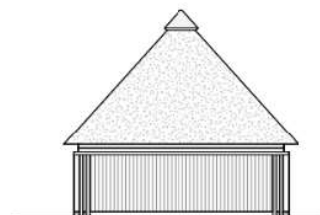
Facade V, laden 1 : 100
