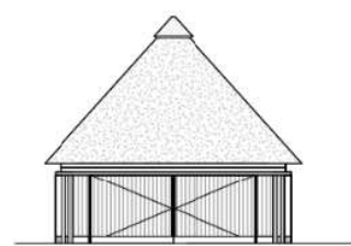
Facade Ø, laden 1 : 100
