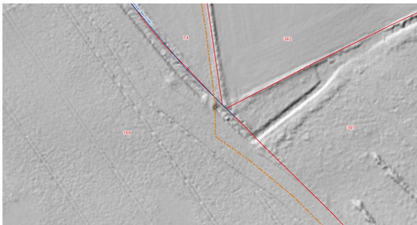
Figur 2: Selskær Bæk, tilløb 2. Råvandsledningen er vist ved orange stiplede linje. Krydsning sker ved underboring
