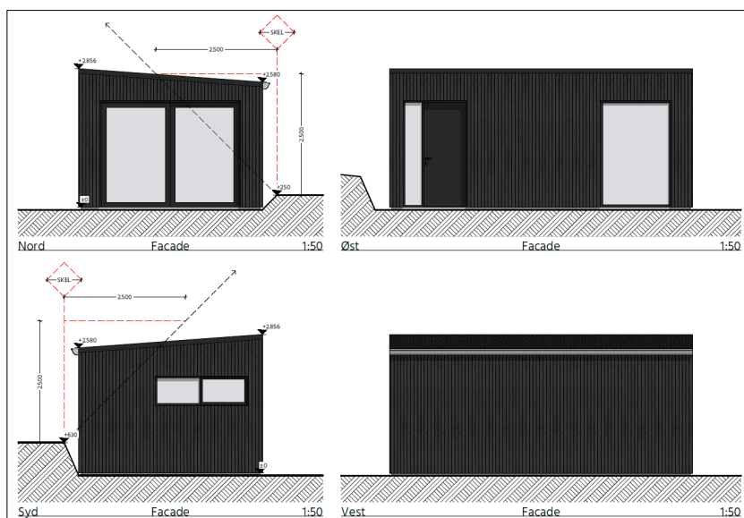
Fra ansøgningen: Facadetegninger
