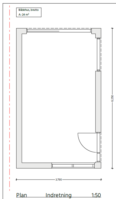
Fra ansøgningen: Plantegningen (målestokken gælder ikke)
