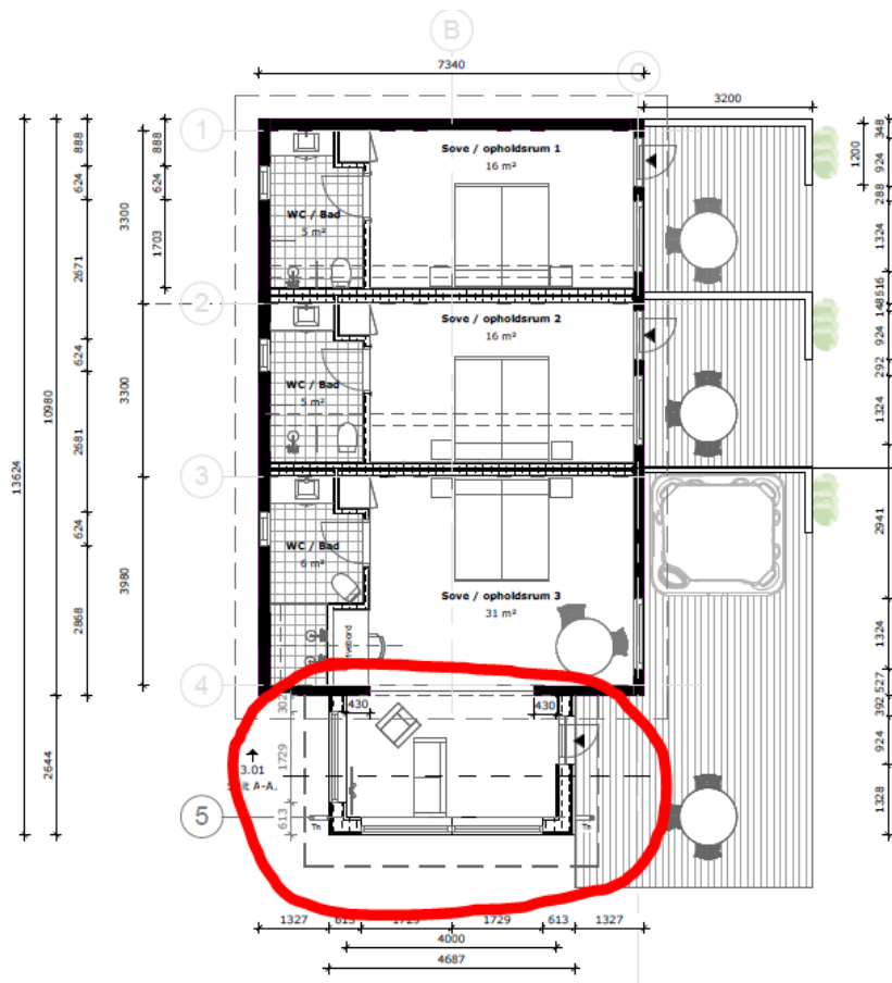
Grundplan med markering af tilbygning
