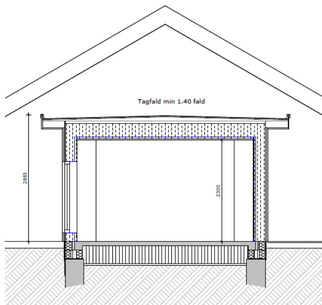
Snit A-A. - 1 : 50
