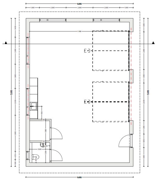
| Plantegning |
